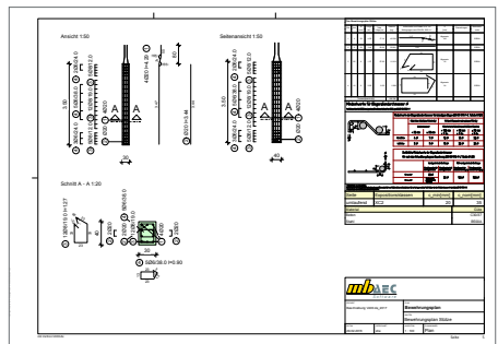
Bewehrungsplan, erstellt mit V400.de
