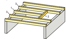
b) Deckenrand
