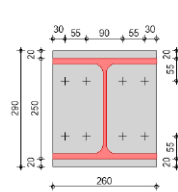
Schnitt A-A
