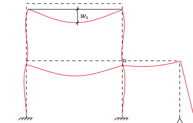
Nachweis Durchbiegung Einzelstäbe
