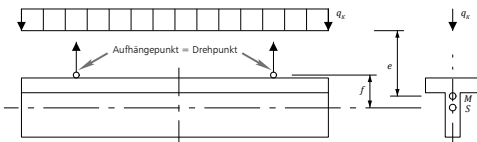
Berechnungsmodell für den kippgefährdeten, aufgehängten Träger nach Lebelte
