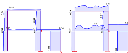
Steifigkeitsverlauf ohne und mit tension stiffening
