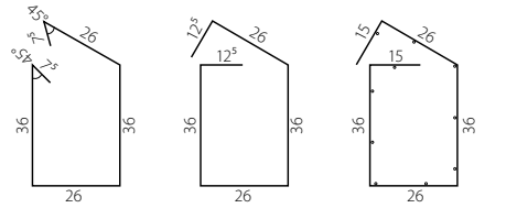
Biegeformen Rechteckbügel
