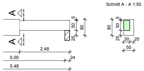
Schalplanausschnitt: Träger mit Querschnittsprung und Versatz
