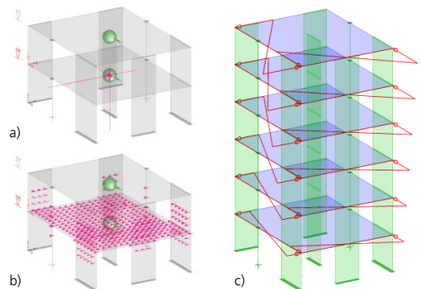
a) Ersatzlasten im selektierten Auswertungsraum b) Konzentrierte Lasten im Lastzentrum c) Zusätzliche Lasten zur nicht planmäßigen Torsionswirkung
