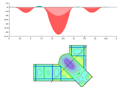
Vergleich Endverformung f_{oo} im Zustand I und Zustand II
