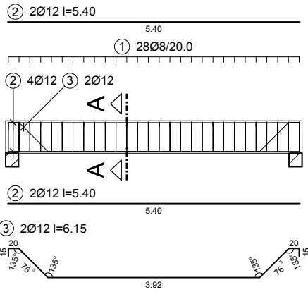
Feldbewehrung mit Schubabiegung
