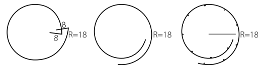
Biegeformen Kreisbügel
