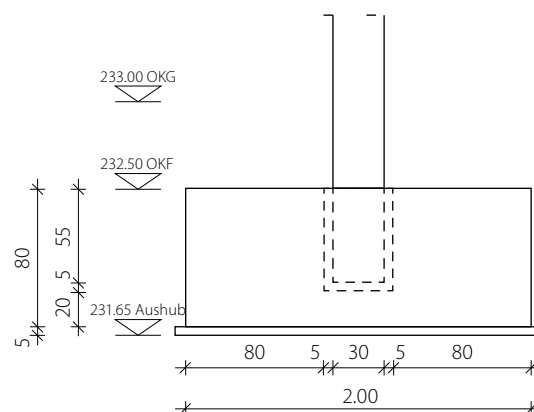
Schalplan Becherfundament mit Höhenkoten
