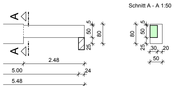
Schalplanausschnitt: Träger mit Querschnittsprung und Versatz
