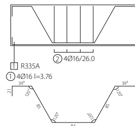
Schnitt Schrägstäbe
