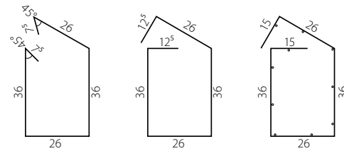
Biegeformen Rechteckbügel
