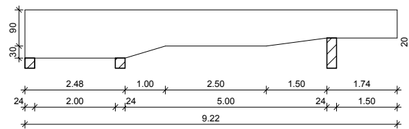
Schalplanausschnitt: mehrfach gevouteter Träger
