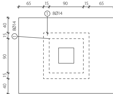
Draufsicht tangentielle Bügelanordnung
