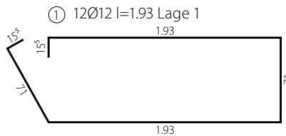
Biegeformen untere Fundamentbewehrung
