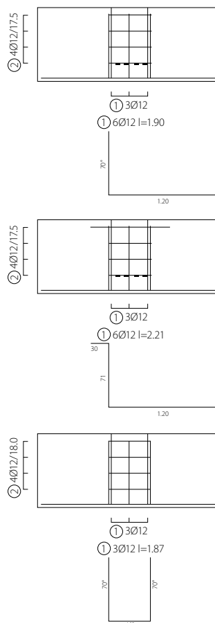
Beispiele Biegeformen Vertikalbügel
