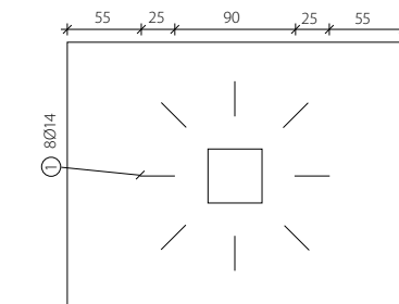
Draufsicht radiale Bügelanordnung
