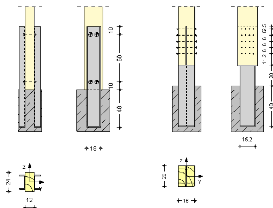
Ausführung mit außenliegenden U-Profilen
