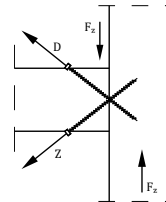
Riegel-Stütze-Anschluss mit gekreuzter Schraubenanordnung:
