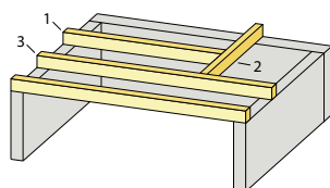
c) Deckenecke
