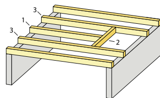
b) Deckenrand
